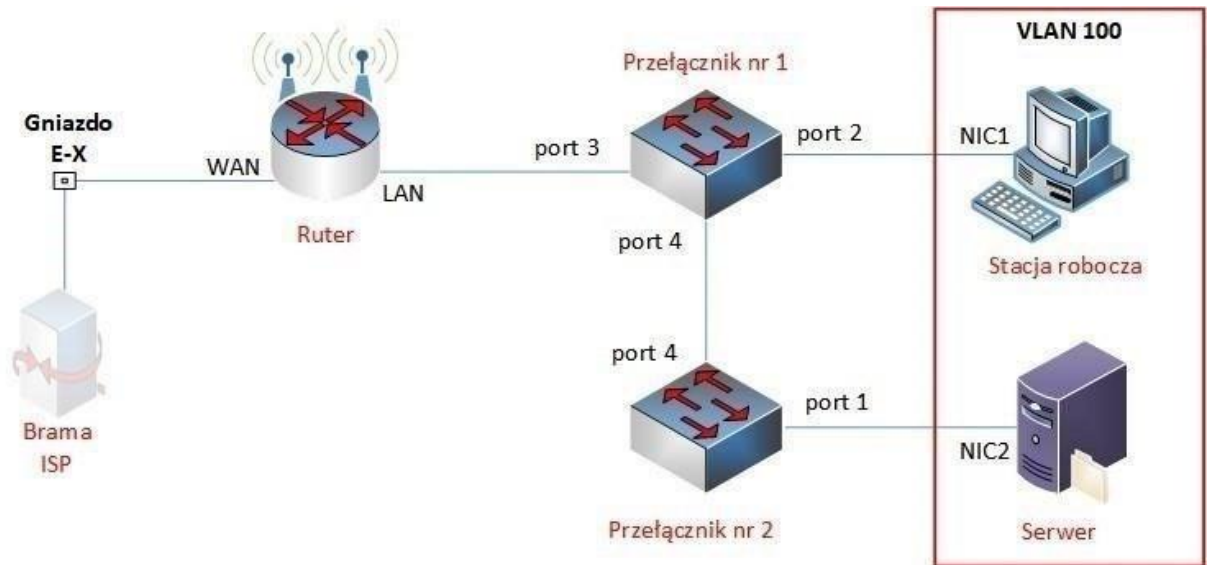
Schemat połączenia urządzeń
